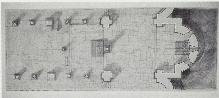
Grundriß der östlichen Michaeliskirche kurz nach dem Tod Bernwards (1022) Rekonstruktion von B. Gallistl/A. Carpiceci
